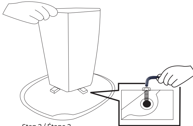
Step 2 / Étape 2 Tighten the Bolts. Visser les boulons, d'abord passés dans un anneau.
